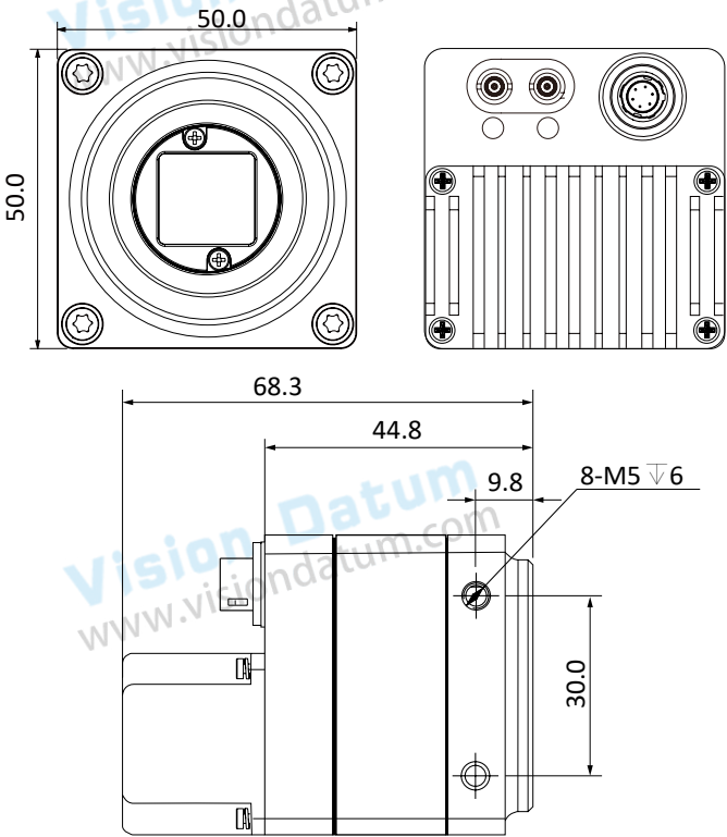
尺寸图
