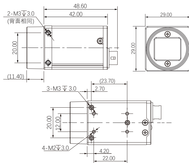
尺寸图
