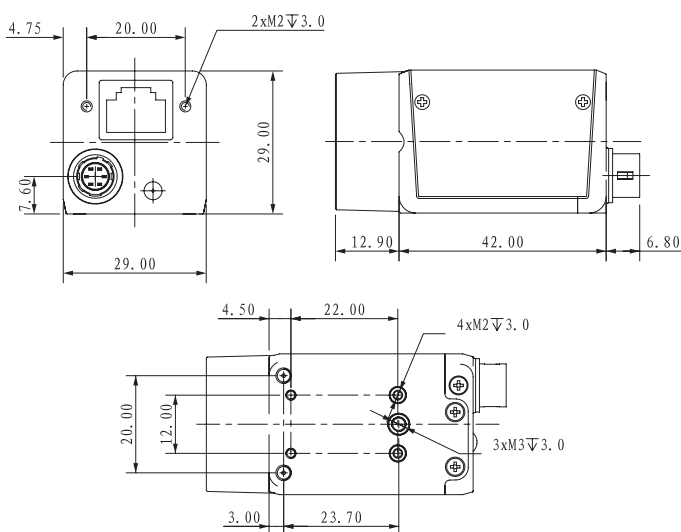
尺寸图
