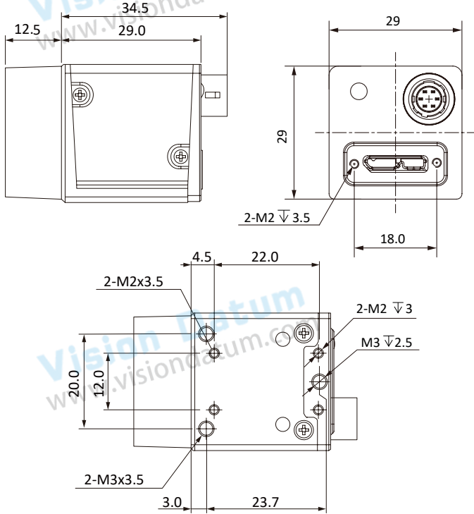
尺寸图
